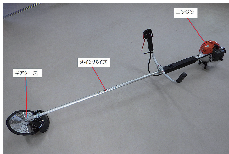
刈払機全景
